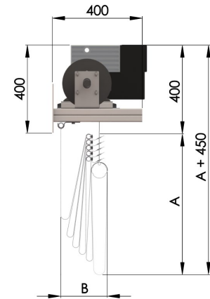
Asennus seinään
