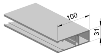
Ohjaukisko 630100
