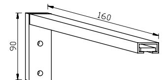
Seinäkannatin 205815
