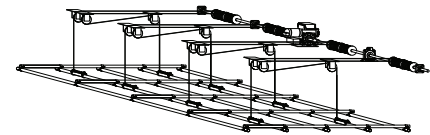
Sähkökäyttöinen putkiristikko 50 mm putkesta PRMK-500. Käytetään lavasteiden, kulissiverhojen ja valaisimien kiinnitykseen. Ristikon maksimikoko 10 x 10 metriä. Putkiristikko voi olla myös kiinteällä kattoasennuksella.
