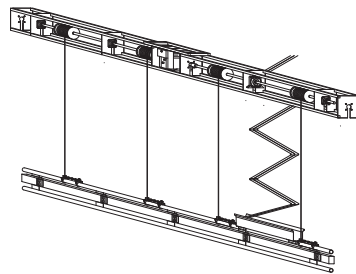
Sähkökäyttöinen valaisinansas ristikolla ja sähköistyspaketilla VMK-250-C
