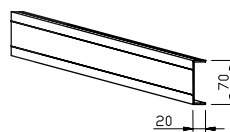
Ramprofil 452070
